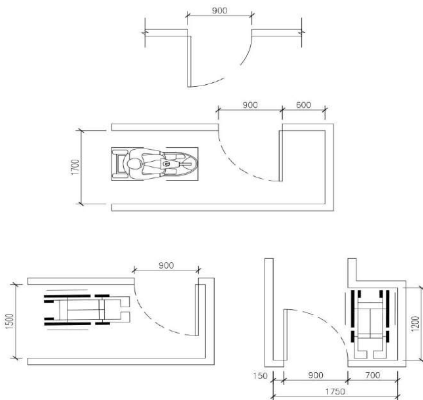
Рис. 9 – Коридори і входи до приміщення
