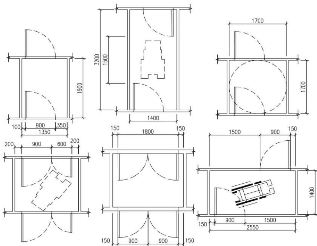
Рис. 8 – Розміри вхідних тамбурів
