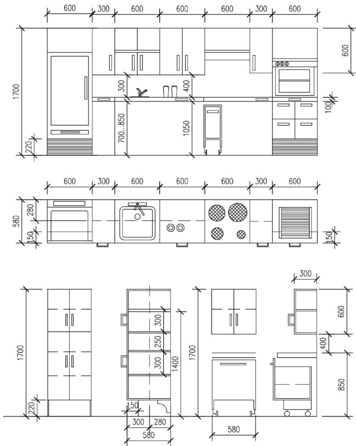
Рис. 18 – Обладнання кухні
