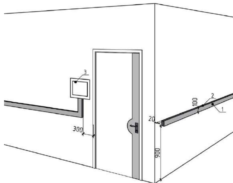
Рис.39 Приклад улаштування тактильних інформаційних позначок приміщень при неможливості розміщення тактильної таблички справа від дверей: 1- інформаційна направляюча, 2- тактильна інформаційна позначка, 3- інформаційна тактильна табличка, що дублює текстову інформацію у тактильному вигляді плоско друкованого тексту та шрифтом Брайля
