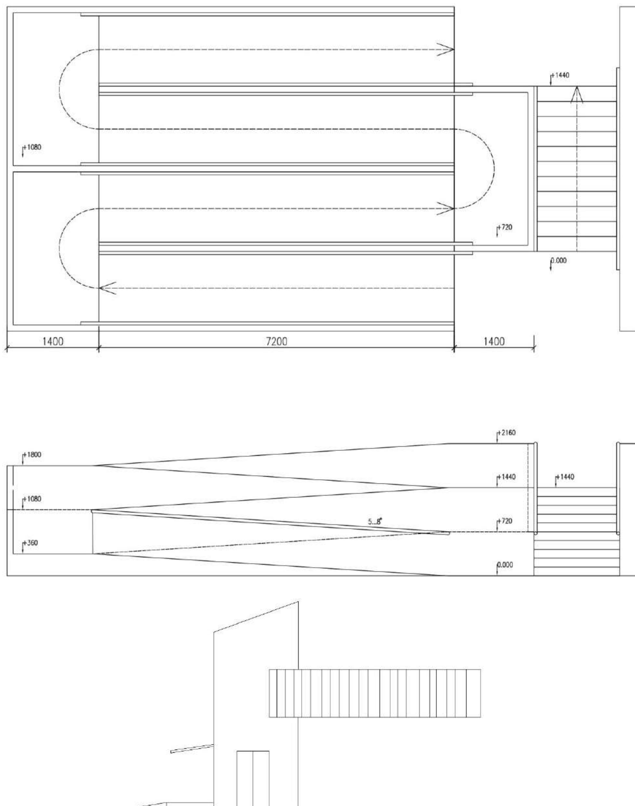
Рис. 3 - Пандус переходу
